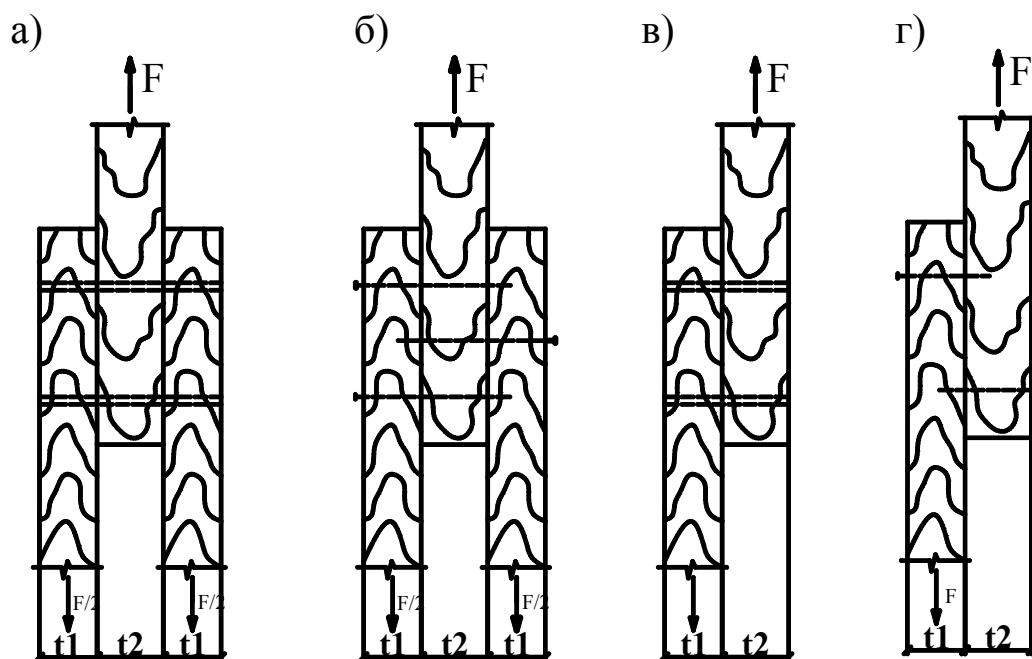
Рисунок 5.1– Соединения древесины с древесиной:
